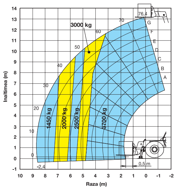
Pe stabilizatoare
