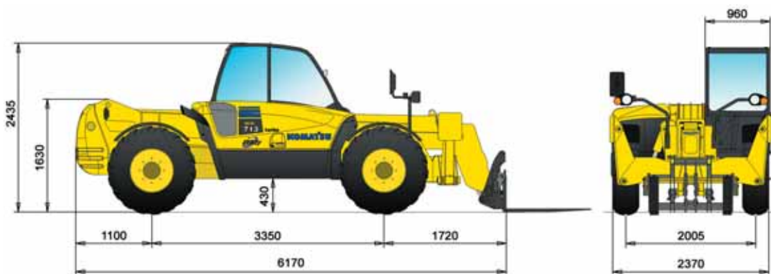
Pe roti
